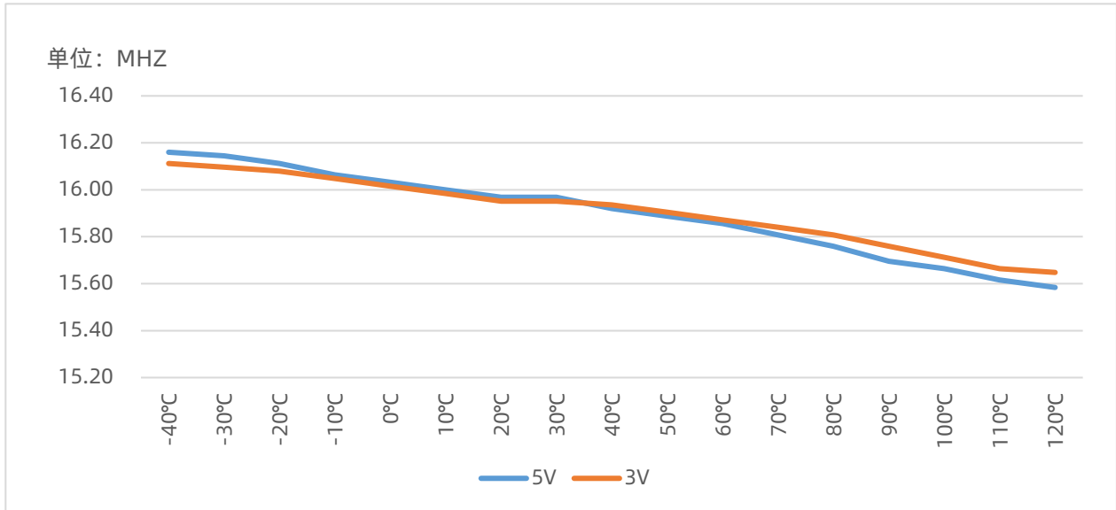
高频时钟（16MHZ）随温度变化典型曲线
