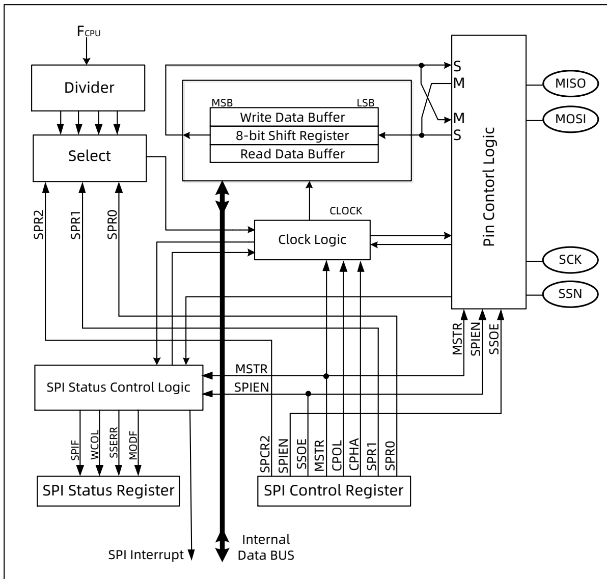
图 12.1 SPI 结构图
