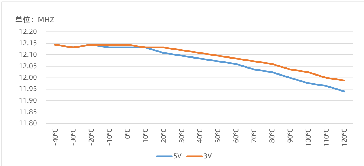
高频时钟（24MHZ）随温度变化典型曲线
