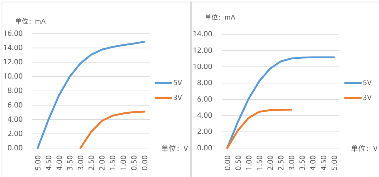
IOH 2 IOL 2
